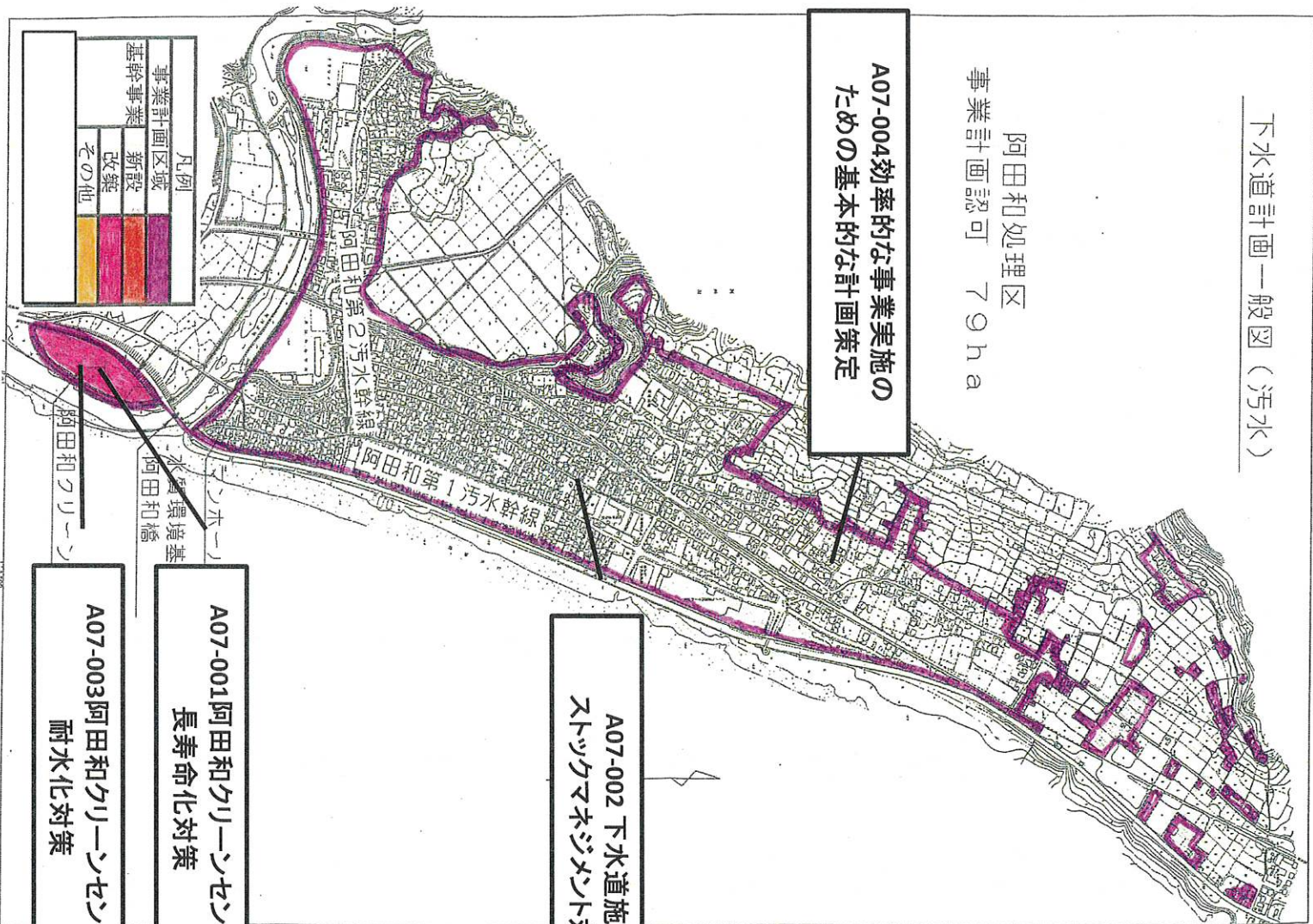
汚水一般平面図
