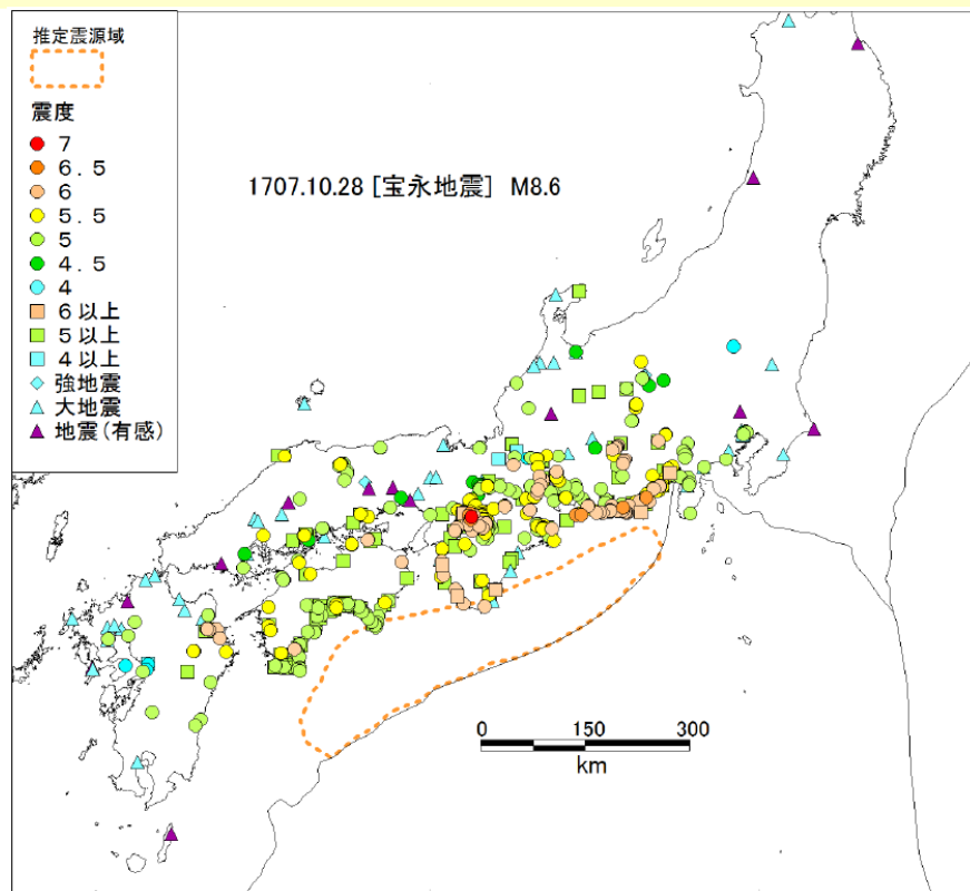
[1707年宝永地震]
