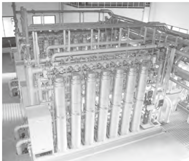
下市木・志原浄水場、阿田和浄水場の高度処理施設
